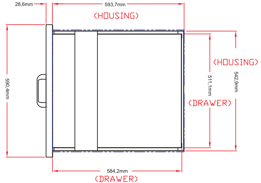
Draufsicht
